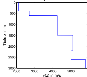
Geschwindigkeitstiefenfunktion
