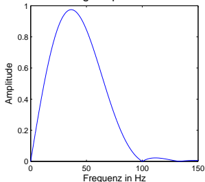
Signalspektrum
