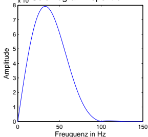
Seismogrammspektrum
