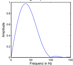
Signalspektrum
