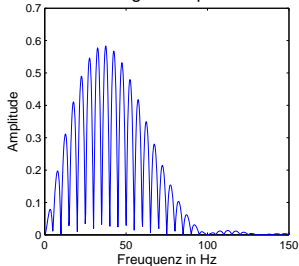
Seismogrammspektrum
